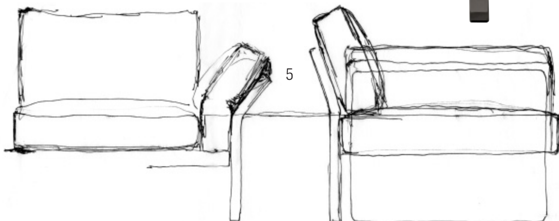
1,3 y 5. Detalles del sofá Metropolitan. Asiento y respaldo reposan sobre una estructura metálica con tiras de piel unidas por hebillas en su parte trasera. 2 y 4. Mesitas Columbus. Tres sobres circulares se combinan.
